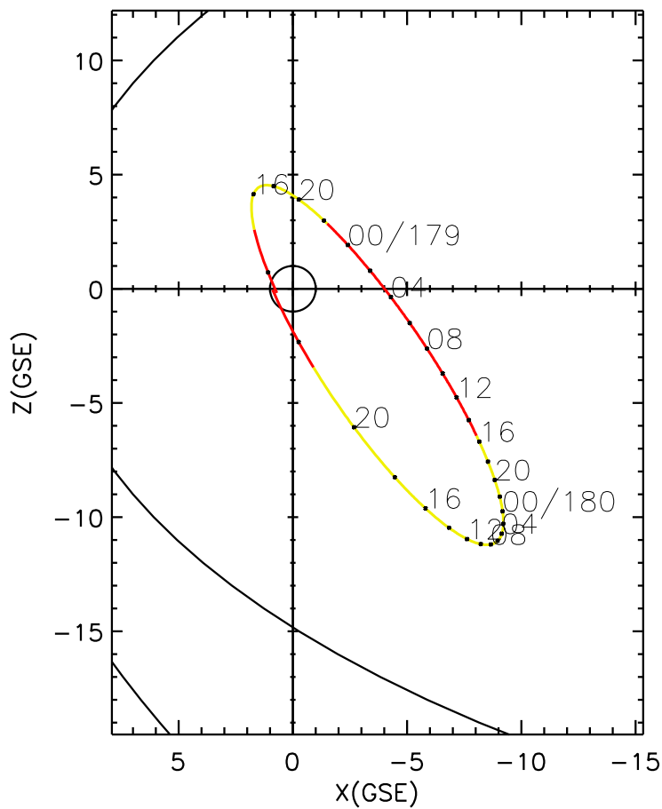
CLUSTER 2 orbit 2007 178 (06/27) 13:41 UT to 2007 180 (06/29) 22:51 UT
