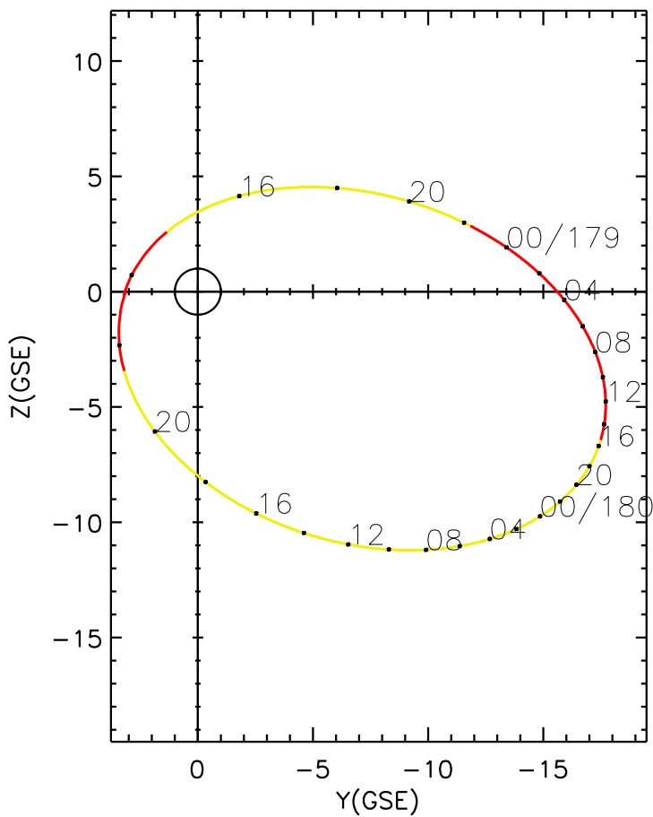
CLUSTER 2 orbit 2007 178 (06/27) 13:41 UT to 2007 180 (06/29) 22:51 UT
