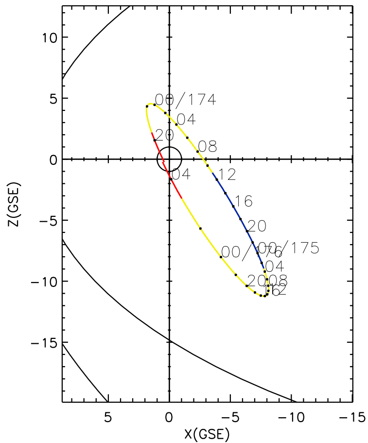
CLUSTER 2 orbit 2007 173 (06/22) 19:21 UT to 2007 176 (06/25) 04:31 UT
