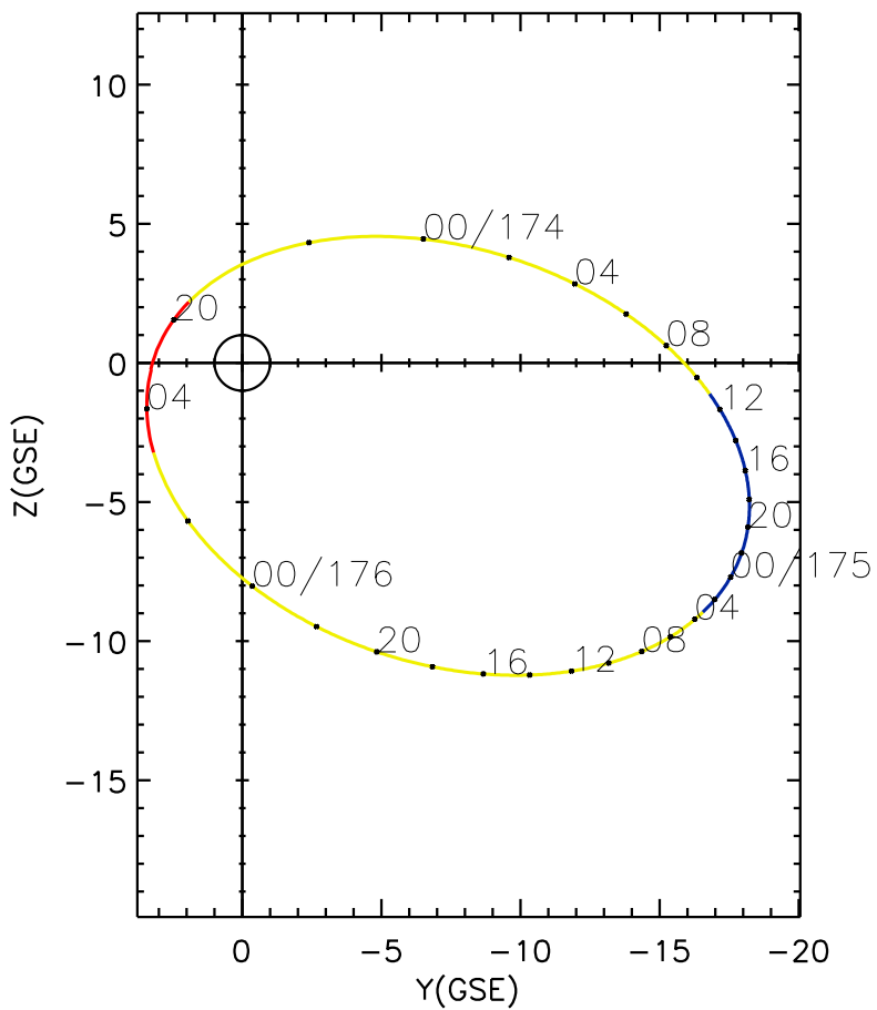
CLUSTER 2 orbit 2007 173 (06/22) 19:21 UT to 2007 176 (06/25) 04:31 UT
