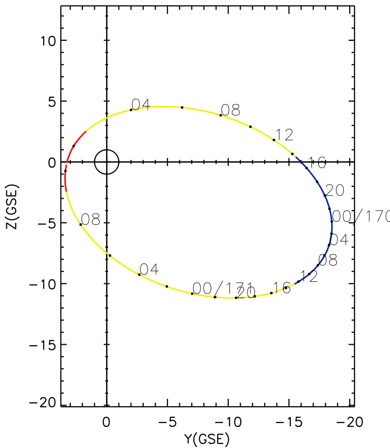
CLUSTER 2 orbit 2007 169 (06/18) 01:31 UT to 2007 171 (06/20) 10:11 UT
