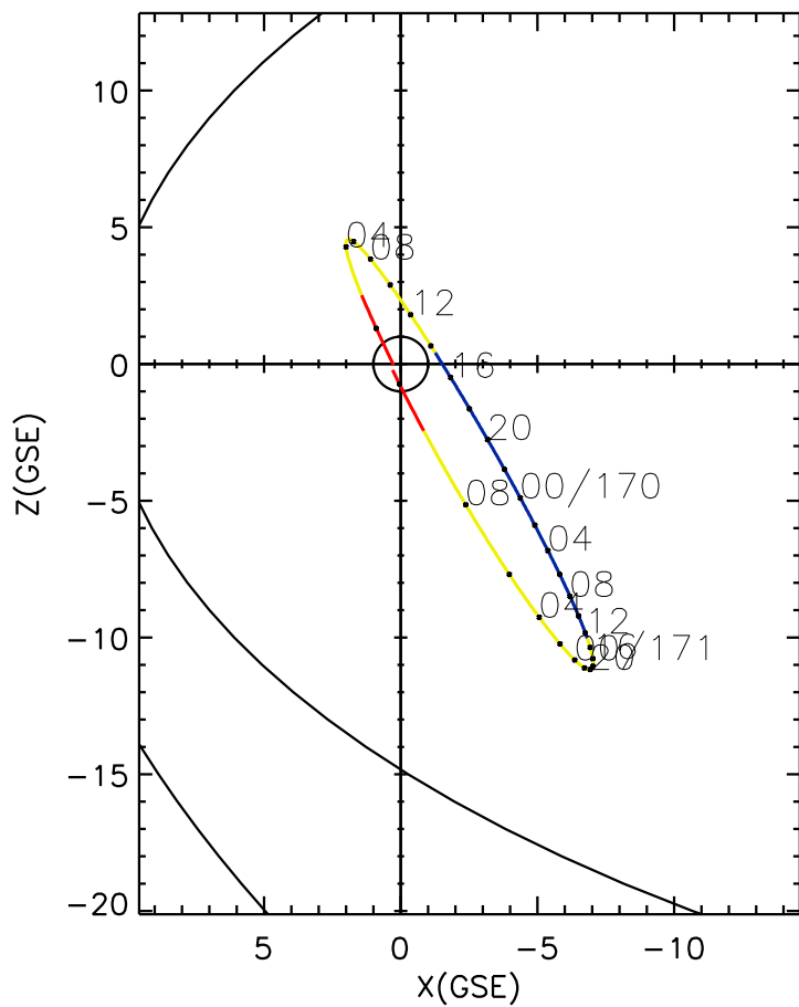
CLUSTER 2 orbit 2007 169 (06/18) 01:31 UT to 2007 171 (06/20) 10:11 UT
