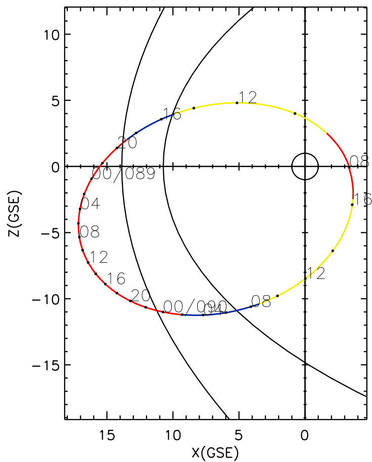
CLUSTER 2 orbit 2007 088 (03/29) 07:56 UT to 2007 090 (03/31) 17:06 UT
