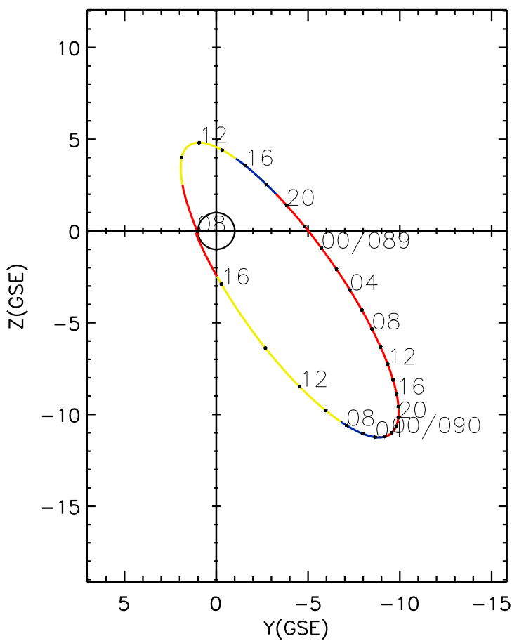
CLUSTER 2 orbit 2007 088 (03/29) 07:56 UT to 2007 090 (03/31) 17:06 UT
