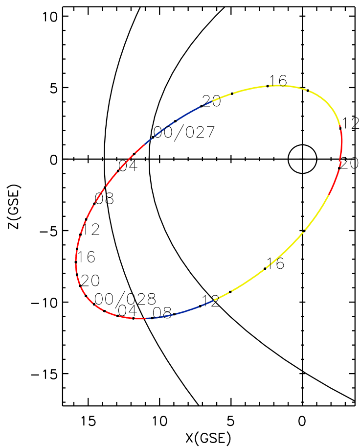
CLUSTER 2 orbit 2007 026 (01/26) 11:06 UT to 2007 028 (01/28) 20:11 UT
