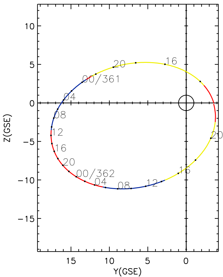
CLUSTER 2 orbit 2006 360 (12/26) 12:51 UT to 2006 362 (12/28) 21:56 UT
