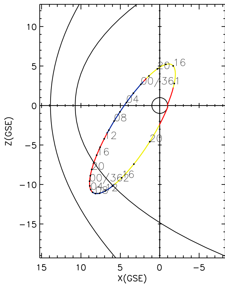
CLUSTER 2 orbit 2006 360 (12/26) 12:51 UT to 2006 362 (12/28) 21:56 UT
