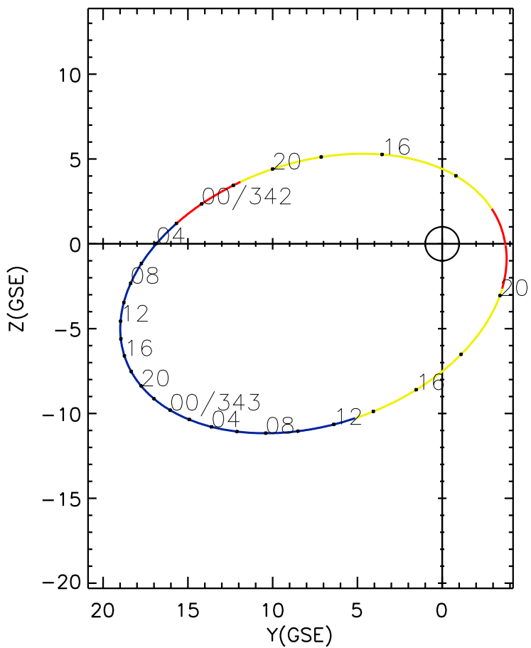
CLUSTER 2 orbit 2006 341 (12/07) 12:06 UT to 2006 343 (12/09) 21:11 UT
