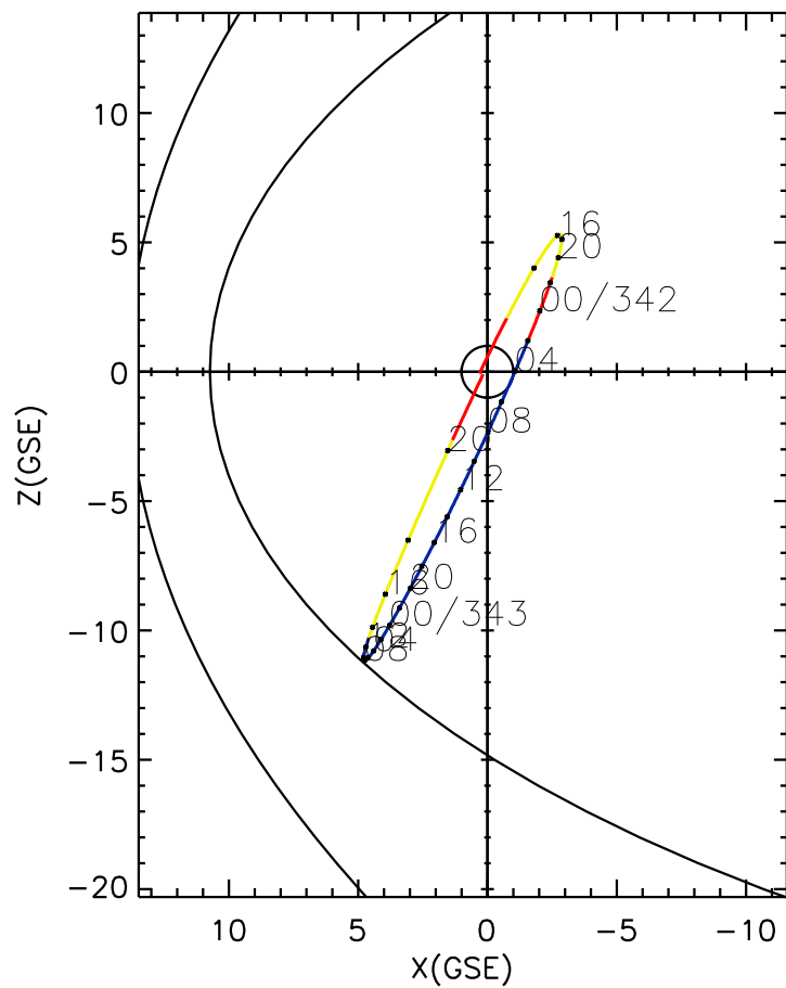
CLUSTER 2 orbit 2006 341 (12/07) 12:06 UT to 2006 343 (12/09) 21:11 UT
