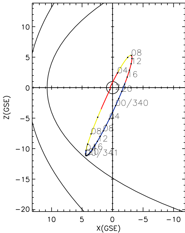
CLUSTER 2 orbit 2006 339 (12/05) 03:01 UT to 2006 341 (12/07) 12:06 UT
