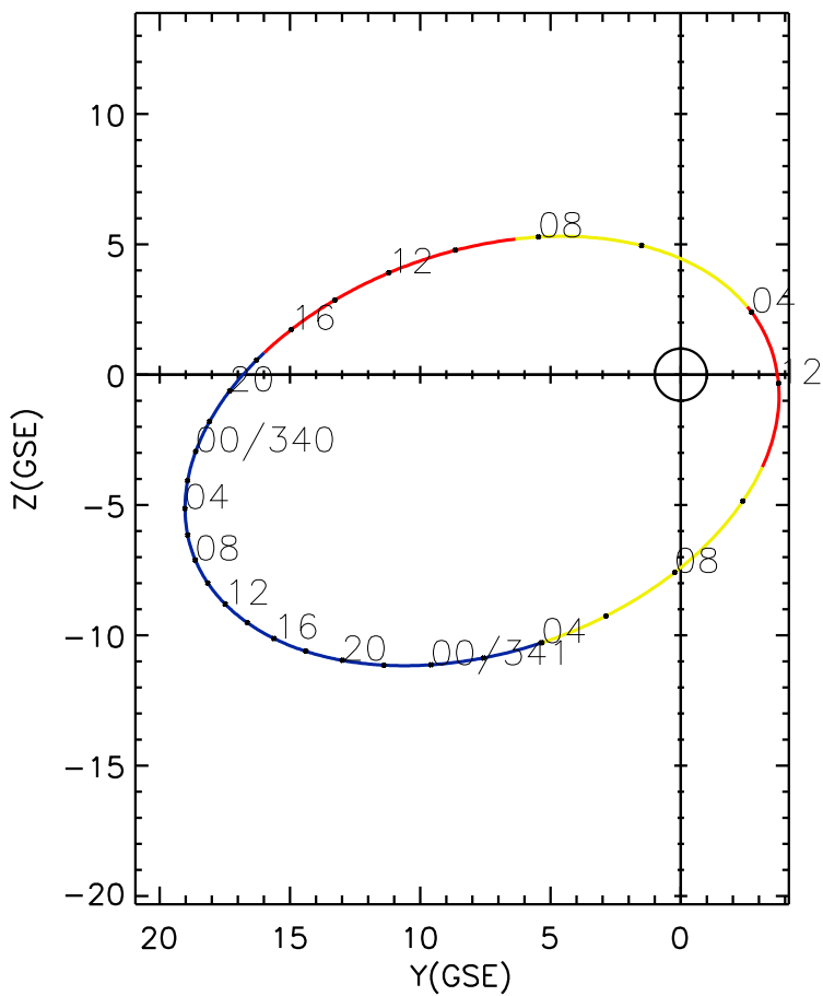
CLUSTER 2 orbit 2006 339 (12/05) 03:01 UT to 2006 341 (12/07) 12:06 UT
