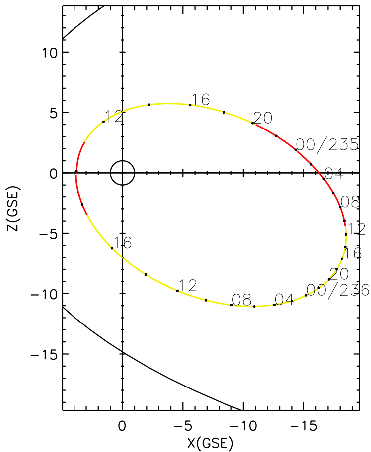
CLUSTER 2 orbit 2006 234 (08/22) 09:56 UT to 2006 236 (08/24) 19:01 UT
