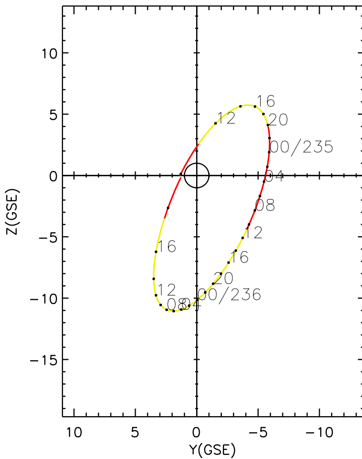
CLUSTER 2 orbit 2006 234 (08/22) 09:56 UT to 2006 236 (08/24) 19:01 UT
