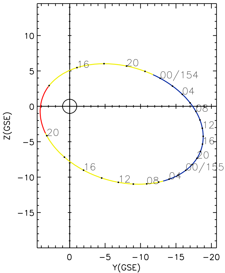
CLUSTER 2 orbit 2006 153 (06/02) 12:41 UT to 2006 155 (06/04) 21:46 UT
