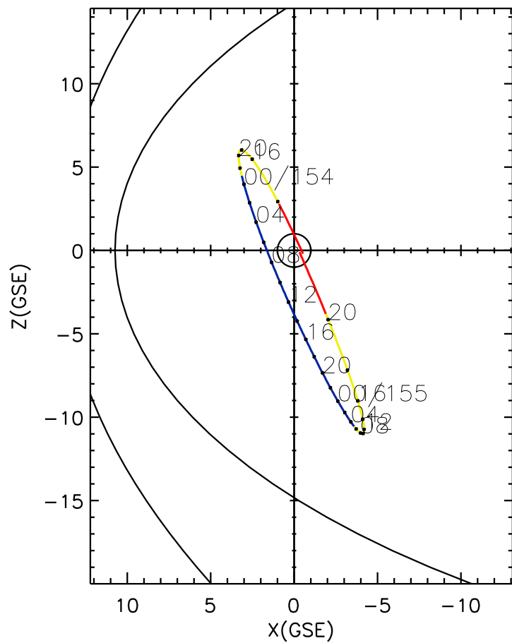
CLUSTER 2 orbit 2006 153 (06/02) 12:41 UT to 2006 155 (06/04) 21:46 UT
