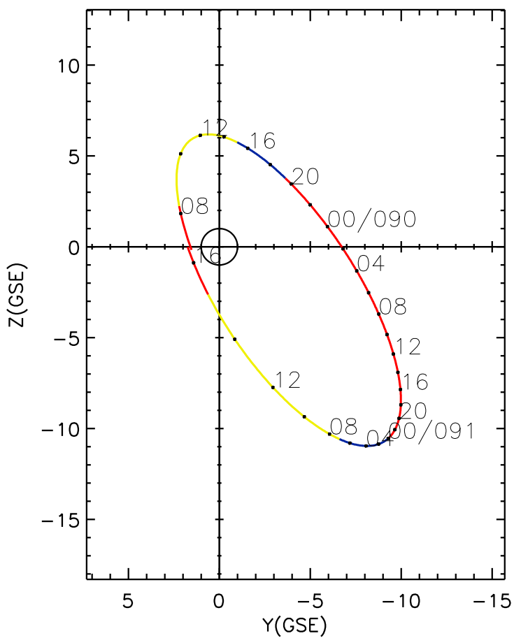
CLUSTER 2 orbit 2006 089 (03/30) 07:11 UT to 2006 091 (04/01) 16:21 UT
