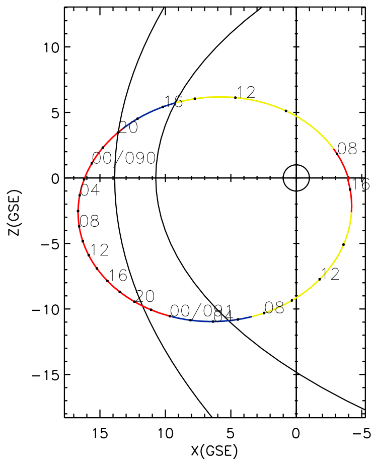
CLUSTER 2 orbit 2006 089 (03/30) 07:11 UT to 2006 091 (04/01) 16:21 UT
