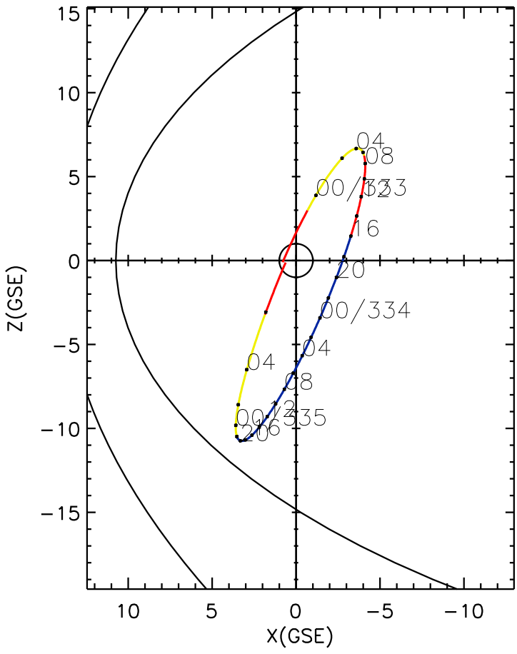
CLUSTER 2 orbit 2005 332 (11/28) 22:11 UT to 2005 335 (12/01) 07:16 UT
