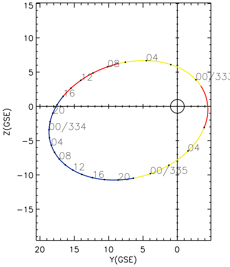
CLUSTER 2 orbit 2005 332 (11/28) 22:11 UT to 2005 335 (12/01) 07:16 UT
