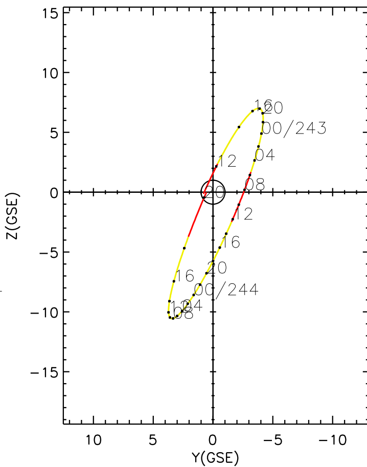
CLUSTER 2 orbit 2005 242 (08/30) 11:01 UT to 2005 244 (09/01) 20:11 UT
