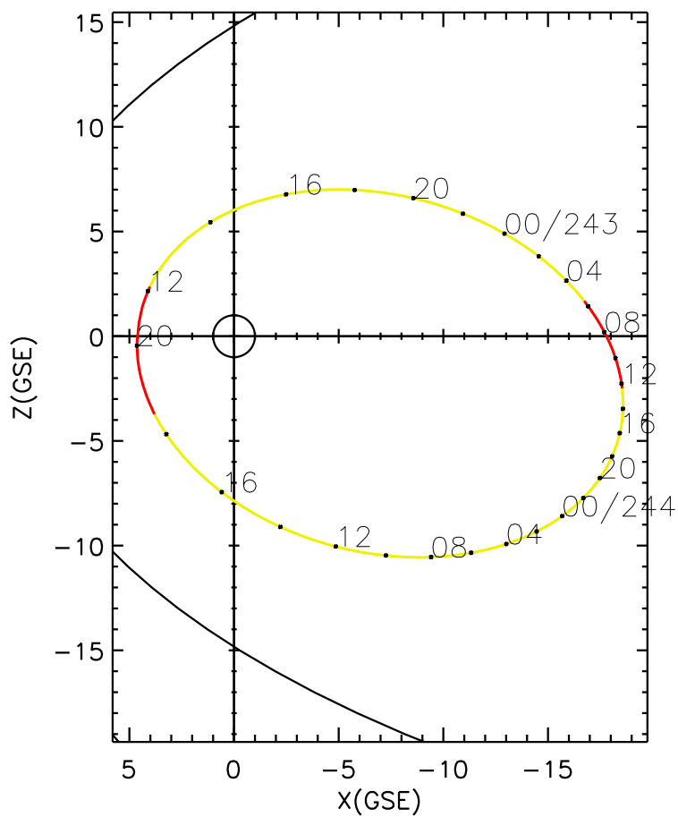
CLUSTER 2 orbit 2005 242 (08/30) 11:01 UT to 2005 244 (09/01) 20:11 UT
