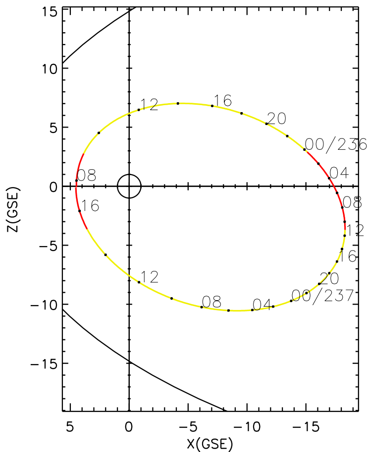
CLUSTER 2 orbit 2005 235 (08/23) 07:46 UT to 2005 237 (08/25) 16:51 UT
