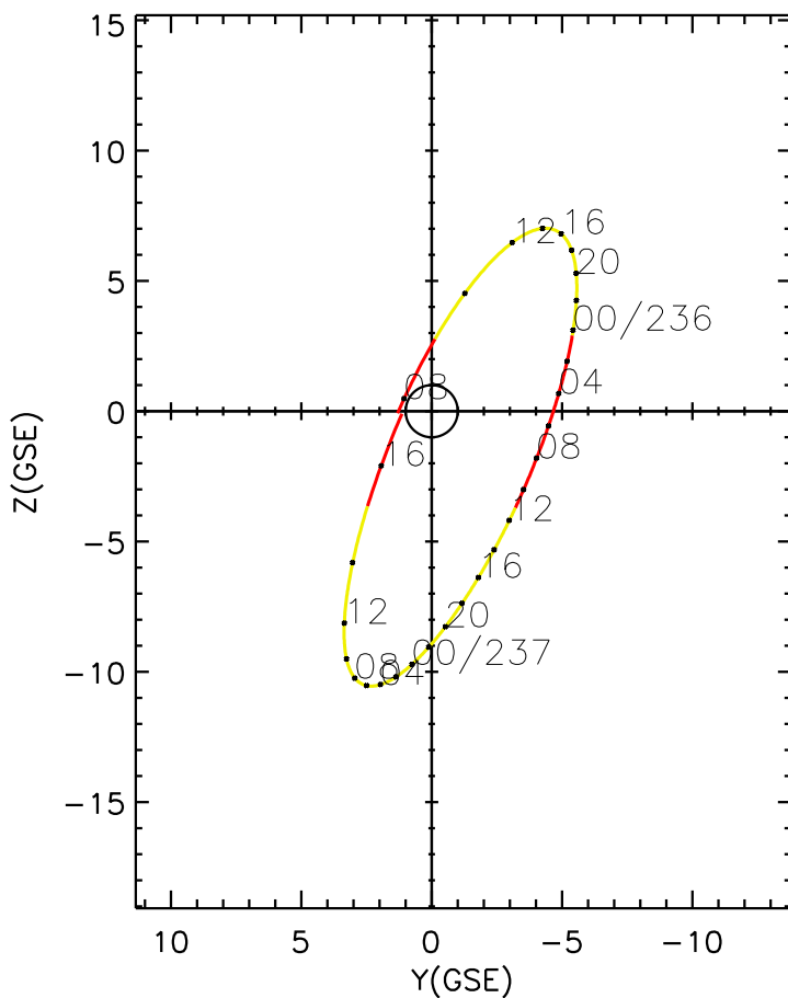
CLUSTER 2 orbit 2005 235 (08/23) 07:46 UT to 2005 237 (08/25) 16:51 UT
