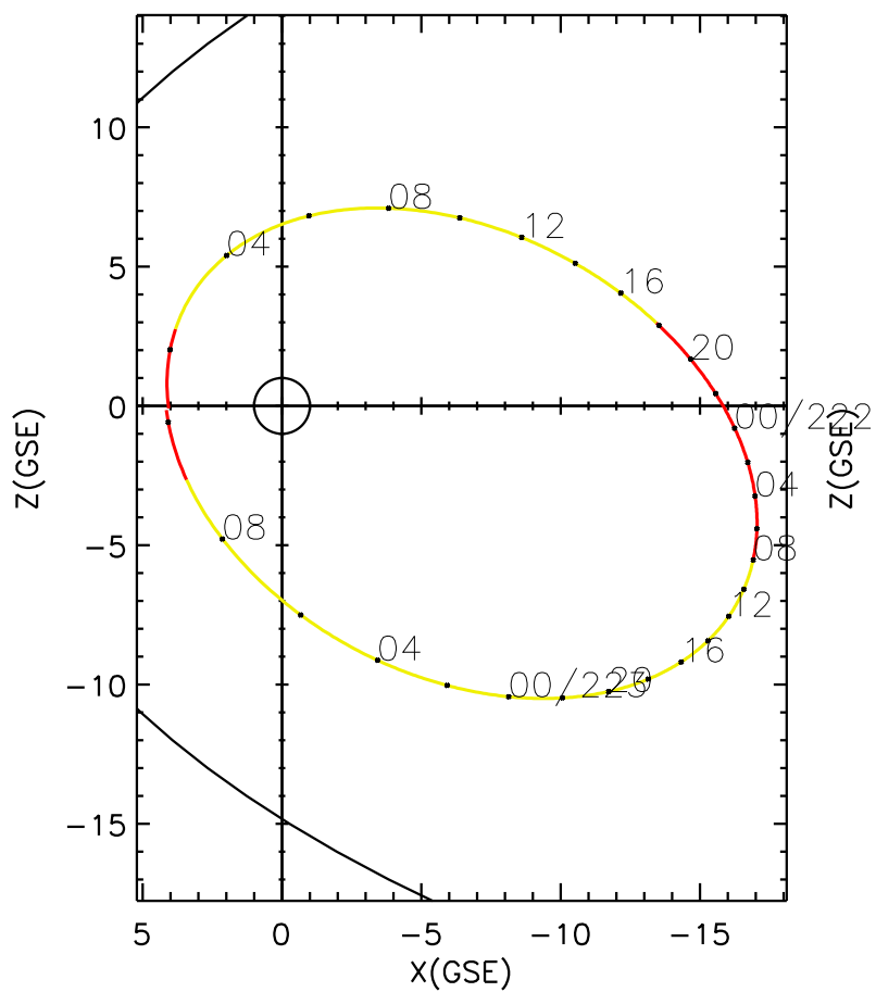
CLUSTER 2 orbit 2005 221 (08/09) 01:06 UT to 2005 223 (08/11) 10:11 UT
