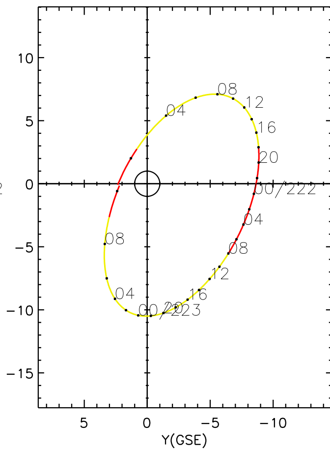
CLUSTER 2 orbit 2005 221 (08/09) 01:06 UT to 2005 223 (08/11) 10:11 UT
