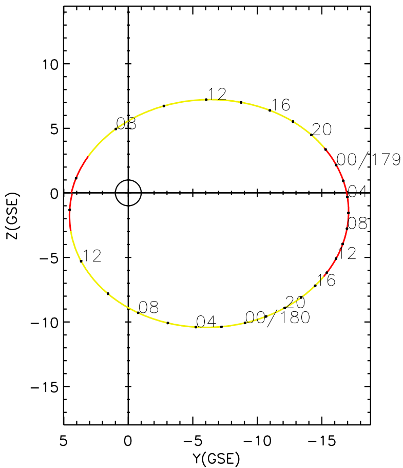
CLUSTER 2 orbit 2005 178 (06/27) 05:31 UT to 2005 180 (06/29) 14:31 UT
