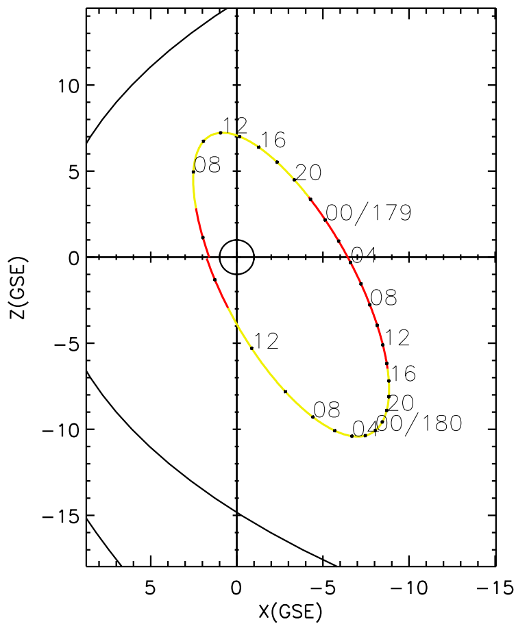
CLUSTER 2 orbit 2005 178 (06/27) 05:31 UT to 2005 180 (06/29) 14:31 UT
