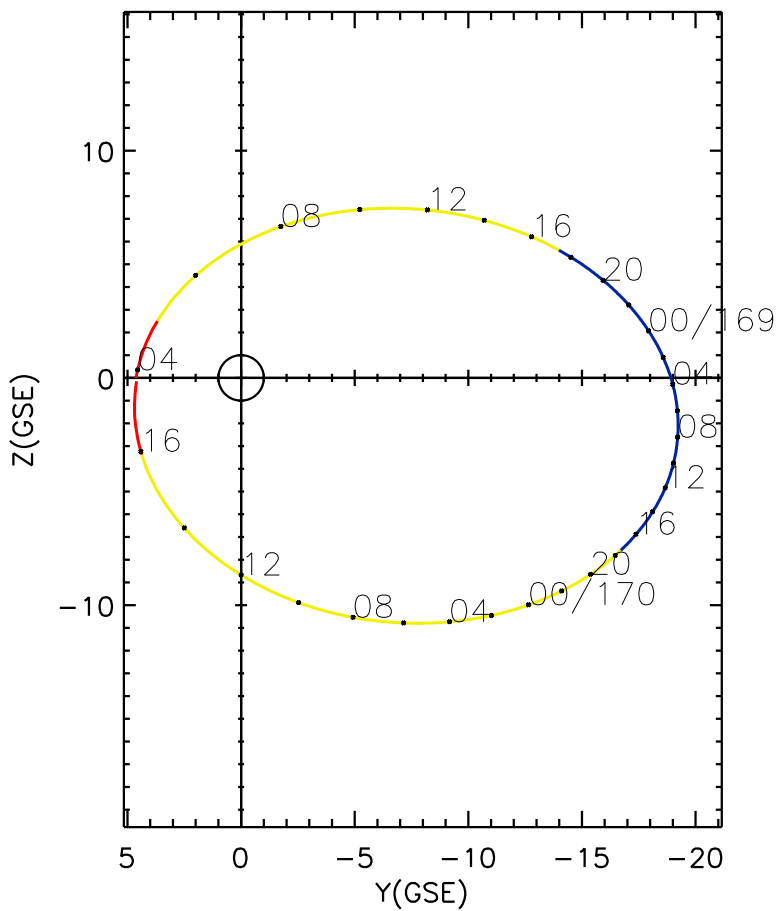
CLUSTER 2 orbit 2005 168 (06/17) 03:51 UT to 2005 170 (06/19) 17:21 UT
