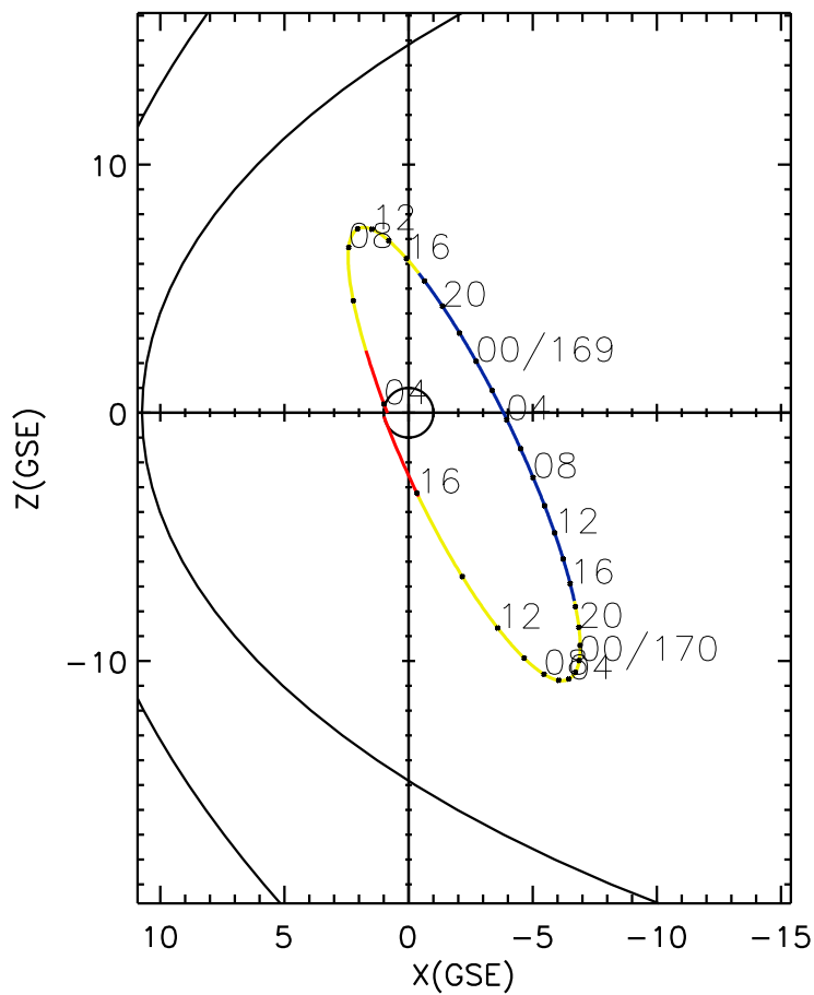
CLUSTER 2 orbit 2005 168 (06/17) 03:51 UT to 2005 170 (06/19) 17:21 UT
