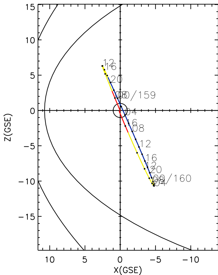
CLUSTER 2 orbit 2005 158 (06/07) 07:16 UT to 2005 160 (06/09) 16:51 UT
