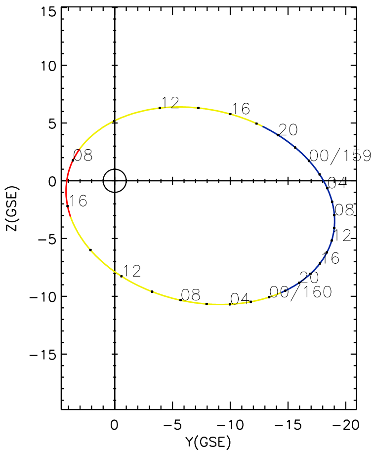
CLUSTER 2 orbit 2005 158 (06/07) 07:16 UT to 2005 160 (06/09) 16:51 UT
