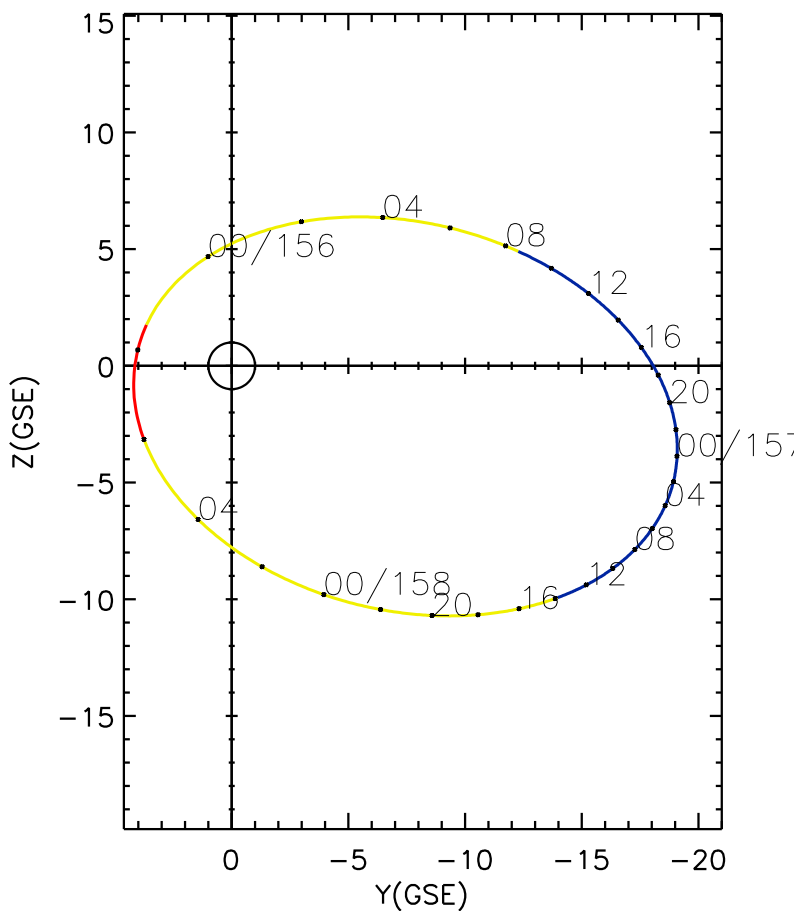
CLUSTER 2 orbit 2005 155 (06/04) 21:41 UT to 2005 158 (06/07) 07:16 UT
