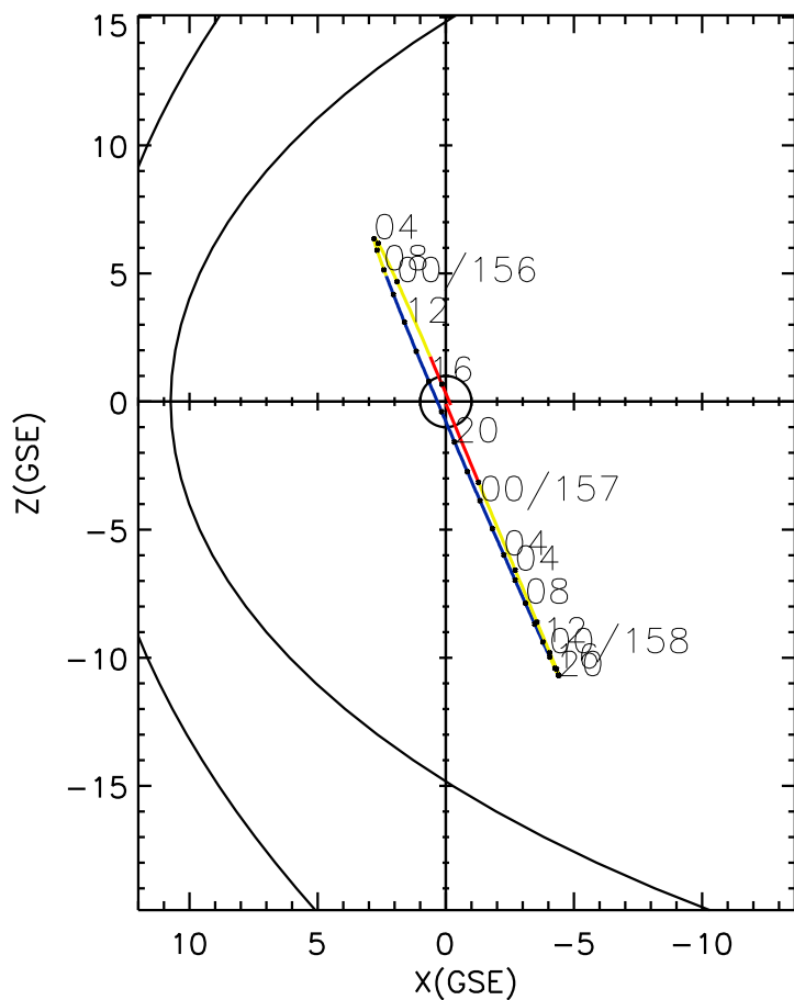
CLUSTER 2 orbit 2005 155 (06/04) 21:41 UT to 2005 158 (06/07) 07:16 UT
