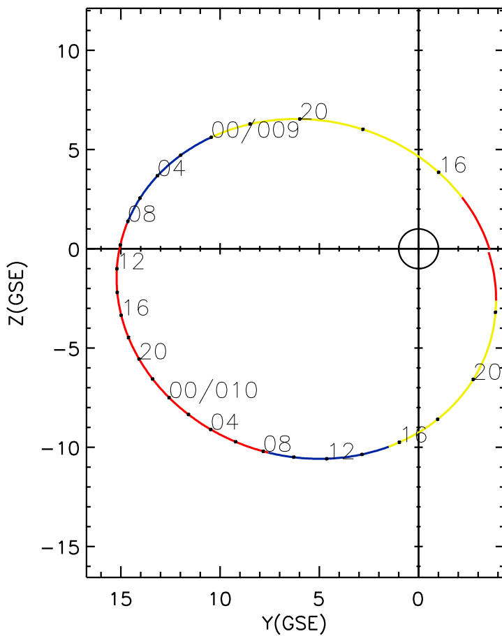
CLUSTER 2 orbit 2005 008 (01/08) 14:16 UT to 2005 010 (01/10) 23:16 UT
