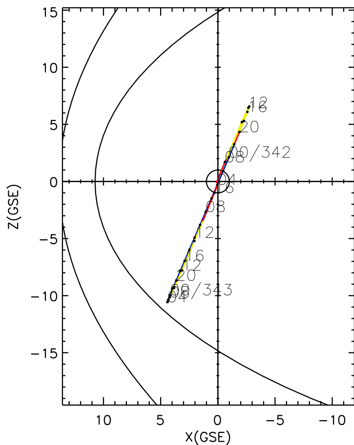
CLUSTER 2 orbit 2004 341 (12/06) 07:16 UT to 2004 343 (12/08) 16:21 UT
