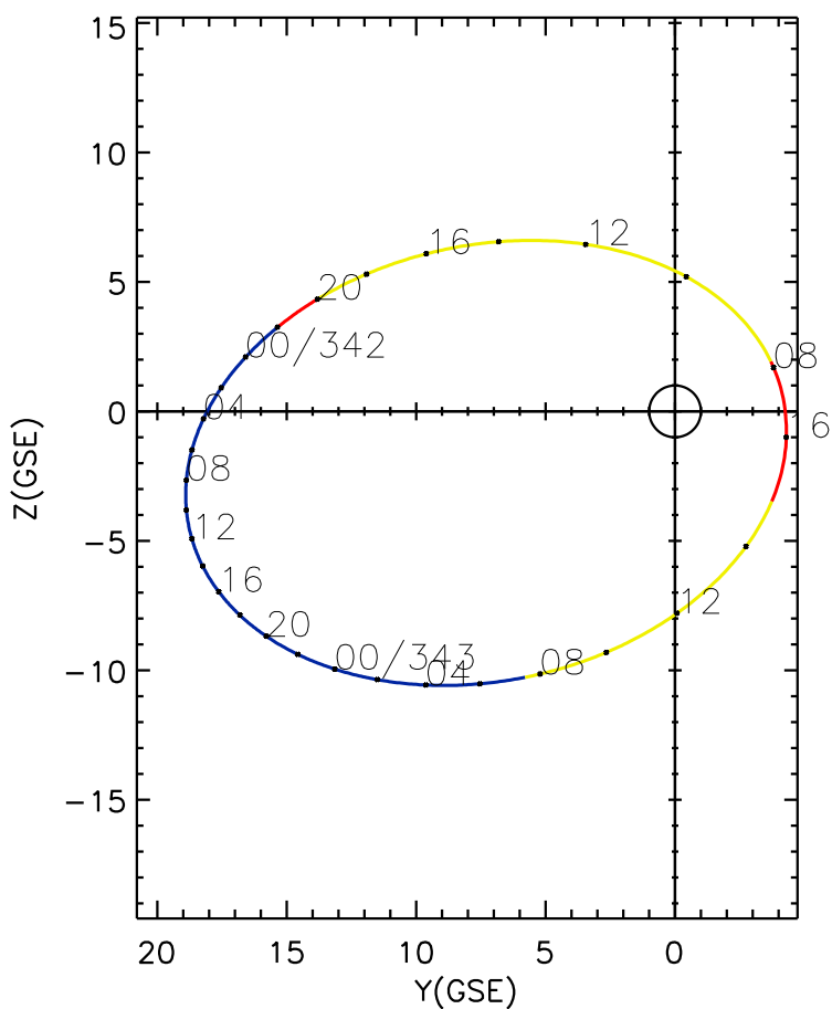
CLUSTER 2 orbit 2004 341 (12/06) 07:16 UT to 2004 343 (12/08) 16:21 UT
