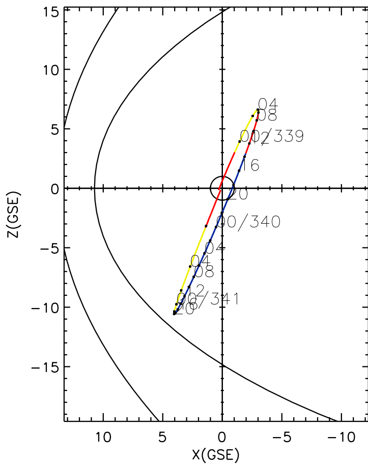
CLUSTER 2 orbit 2004 338 (12/03) 22:11 UT to 2004 341 (12/06) 07:16 UT
