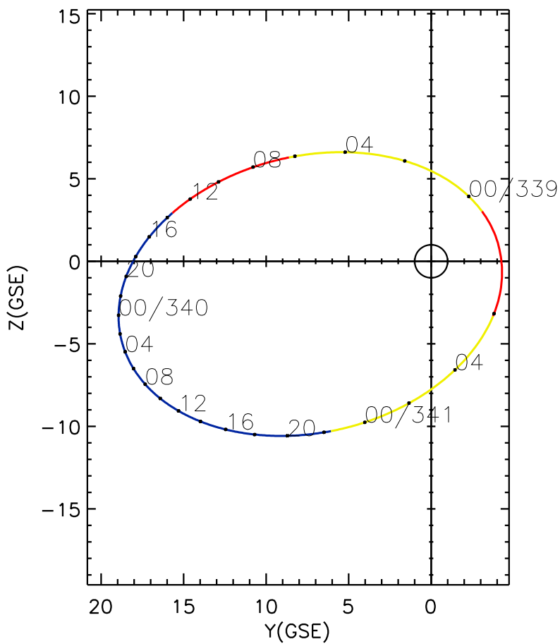
CLUSTER 2 orbit 2004 338 (12/03) 22:11 UT to 2004 341 (12/06) 07:16 UT
