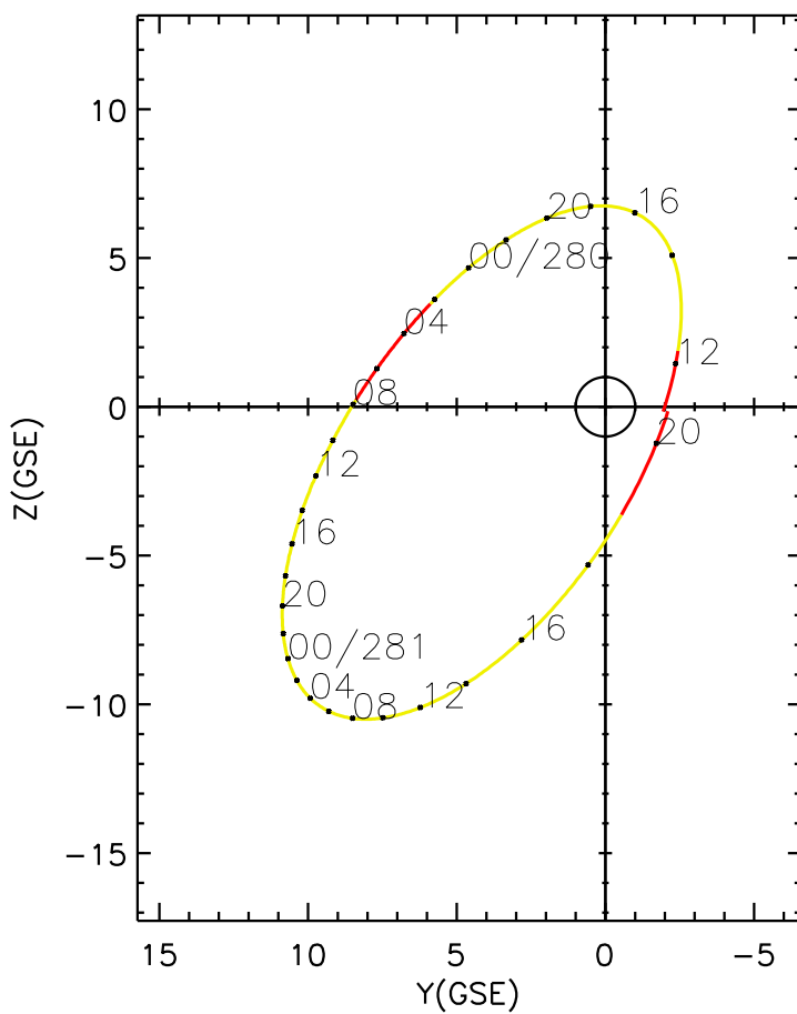
CLUSTER 2 orbit 2004 279 (10/05) 11:21 UT to 2004 281 (10/07) 20:26 UT
