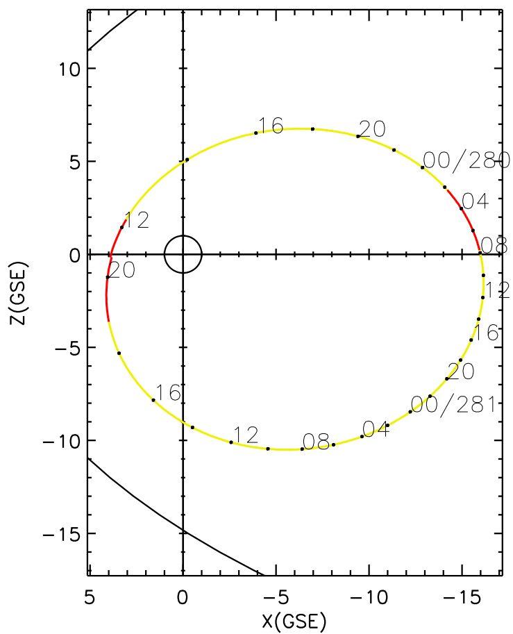
CLUSTER 2 orbit 2004 279 (10/05) 11:21 UT to 2004 281 (10/07) 20:26 UT
