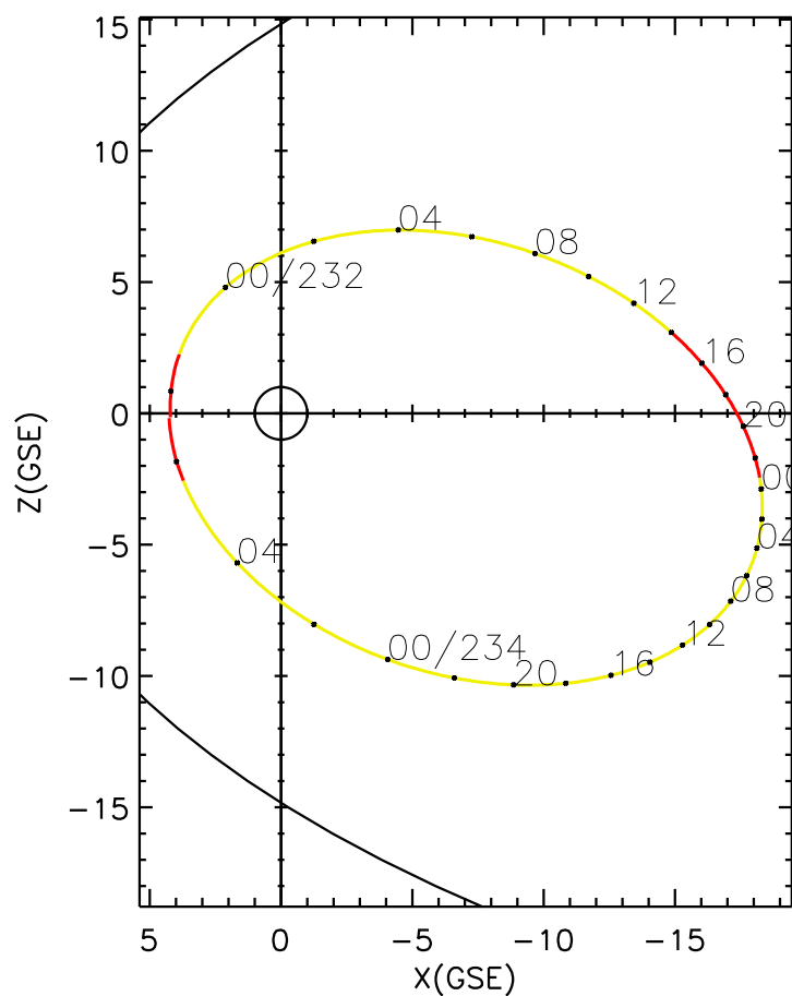
CLUSTER 2 orbit 2004 231 (08/18) 21:36 UT to 2004 234 (08/21) 06:41 UT
