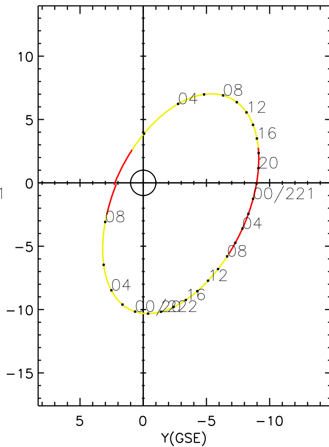
CLUSTER 2 orbit 2004 220 (08/07) 00:11 UT to 2004 222 (08/09) 09:16 UT
