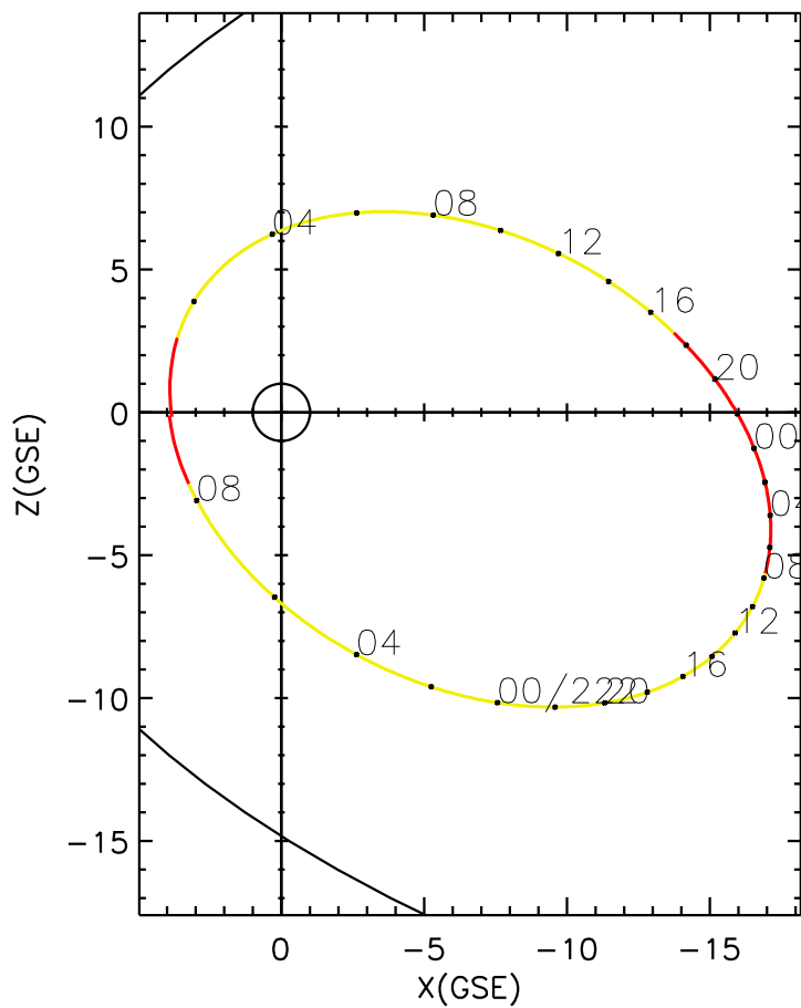
CLUSTER 2 orbit 2004 220 (08/07) 00:11 UT to 2004 222 (08/09) 09:16 UT
