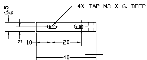
PART -02 QTY 2 PER ASSY
