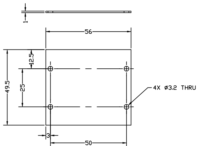
PART -03 QTY 1 PER ASSY
