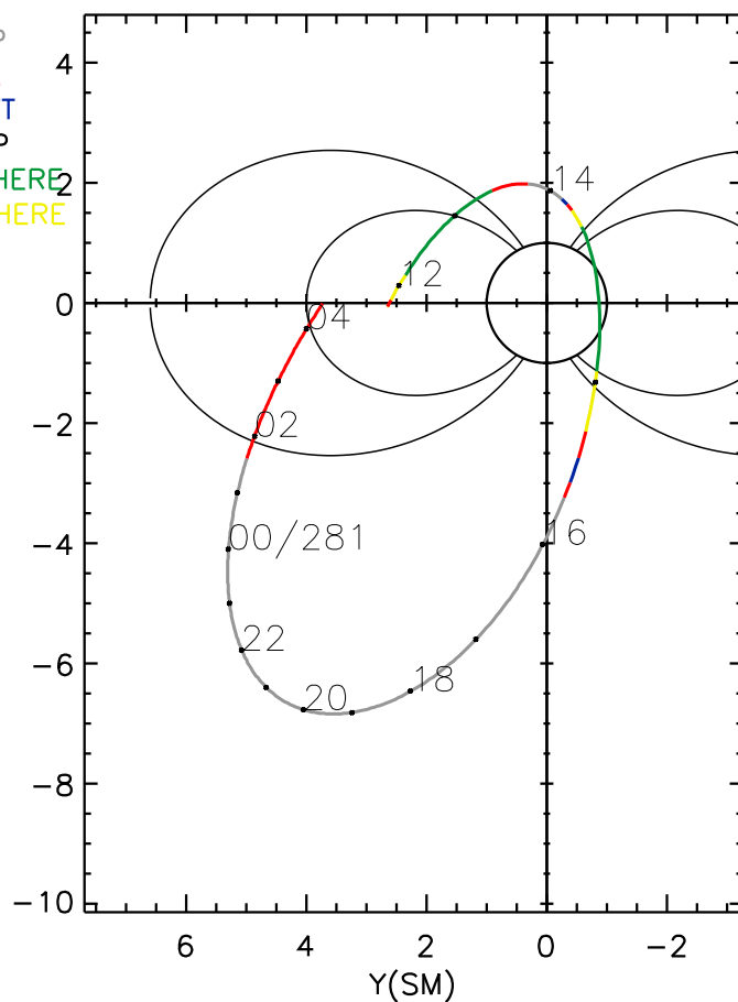
POLAR orbit 2004 280 (10/06) 11:42 UT to 2004 281 (10/07) 04:30 UT
