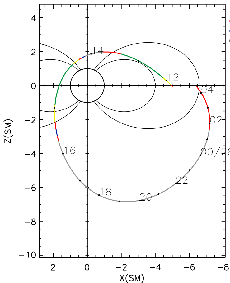
POLAR orbit 2004 280 (10/06) 11:42 UT to 2004 281 (10/07) 04:30 UT
