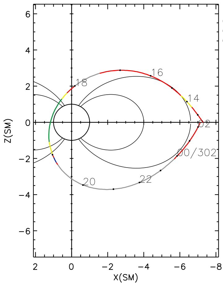
POLAR orbit 2002 301 (10/28) 12:21 UT to 2002 302 (10/29) 02:21 UT
