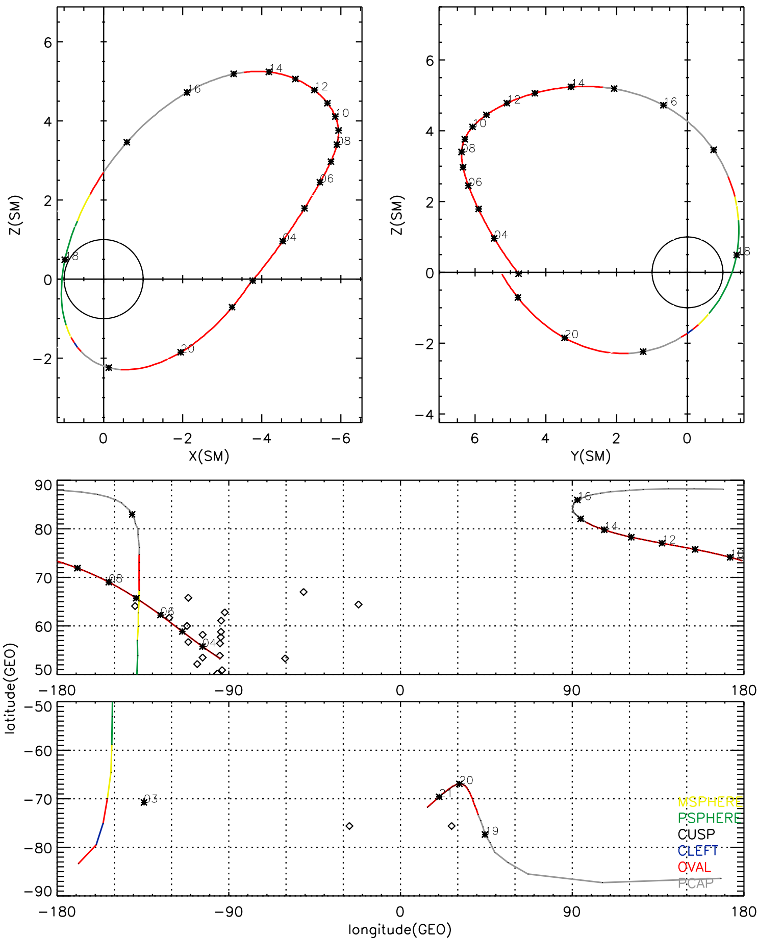
POLAR orbit 2000 325 (11/20) 03:00 UT to 2000 325 (11/20) 21:30 UT
