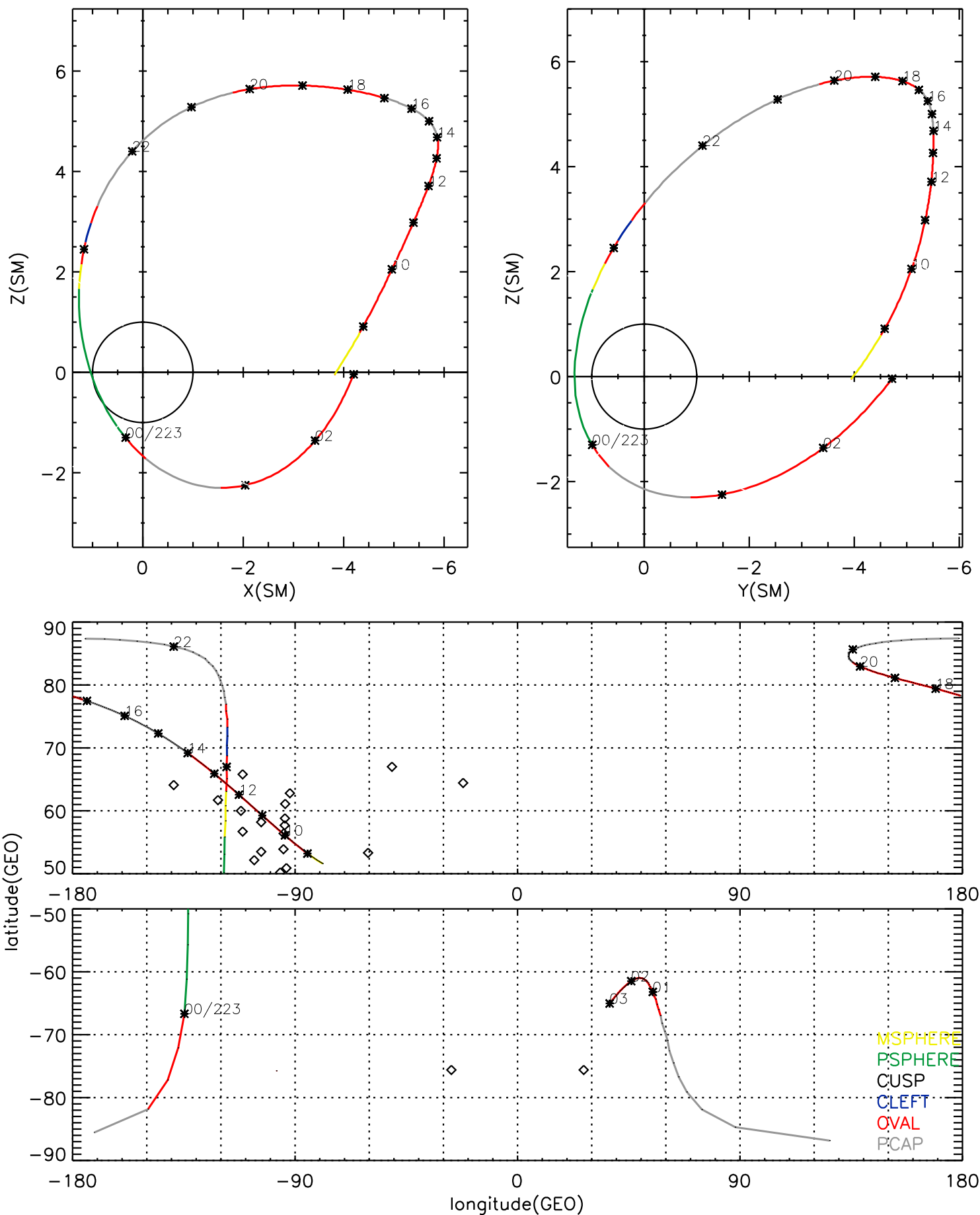
POLAR orbit 2000 222 (08/09) 08:15 UT to 2000 223 (08/10) 03:00 UT
