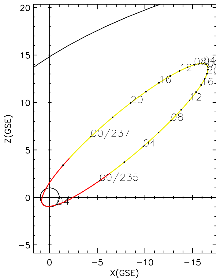
CLUSTER 2 orbit 2024 234 (08/21) 22:21 UT to 2024 237 (08/24) 04:36 UT
