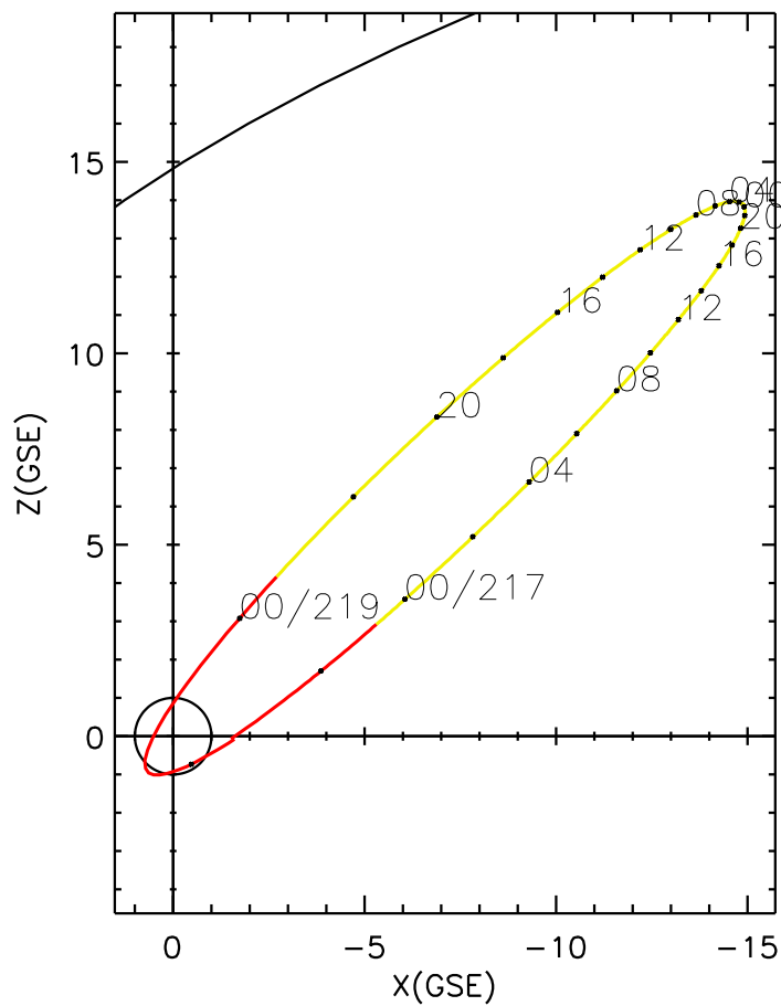
CLUSTER 2 orbit 2024 216 (08/03) 20:21 UT to 2024 219 (08/06) 02:36 UT
