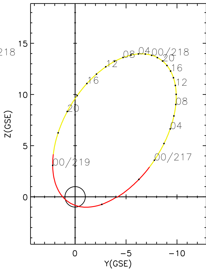
CLUSTER 2 orbit 2024 216 (08/03) 20:21 UT to 2024 219 (08/06) 02:36 UT
