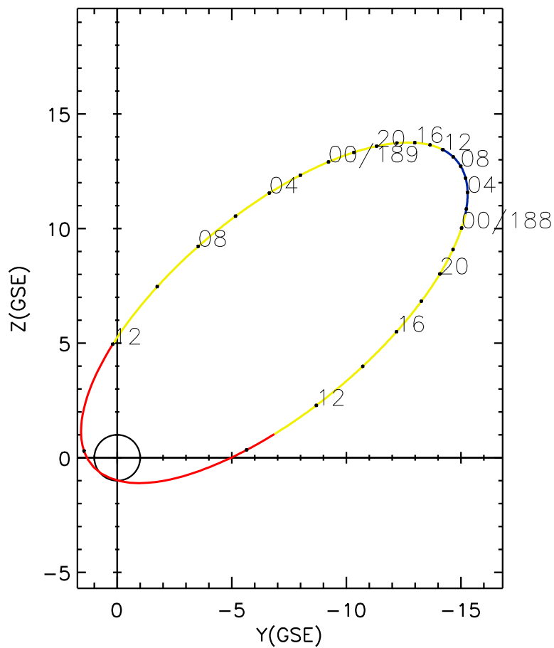
CLUSTER 2 orbit 2024 187 (07/05) 09:36 UT to 2024 189 (07/07) 15:51 UT
