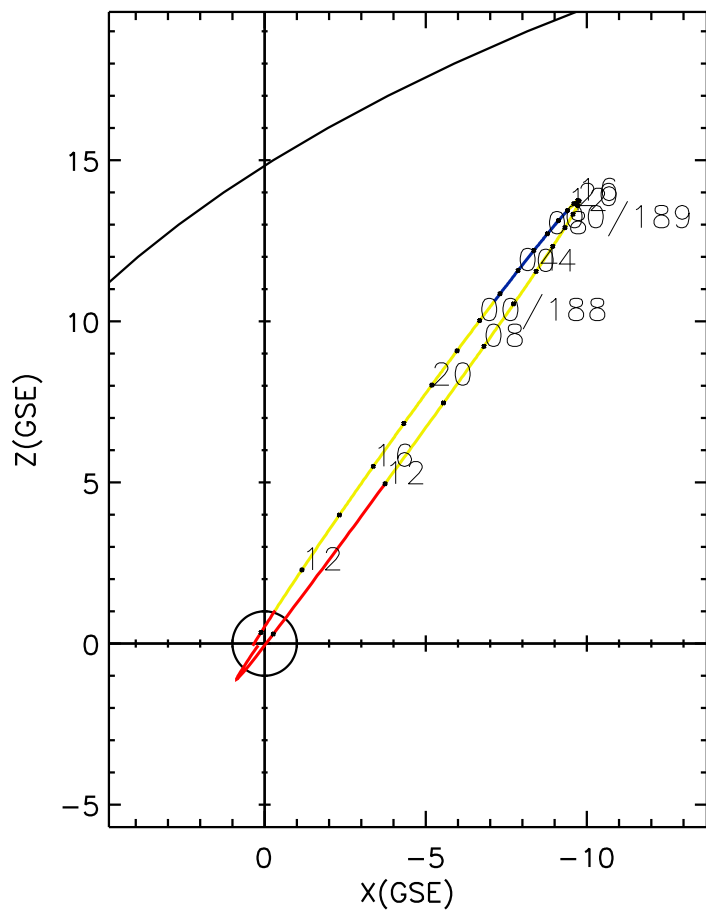
CLUSTER 2 orbit 2024 187 (07/05) 09:36 UT to 2024 189 (07/07) 15:51 UT
