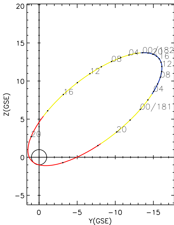
CLUSTER 2 orbit 2024 180 (06/28) 16:26 UT to 2024 182 (06/30) 22:41 UT
