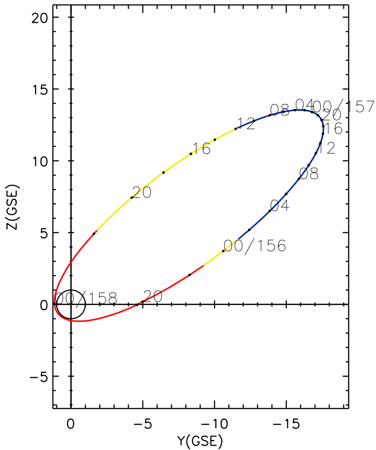
CLUSTER 2 orbit 2024 155 (06/03) 19:46 UT to 2024 158 (06/06) 02:01 UT
