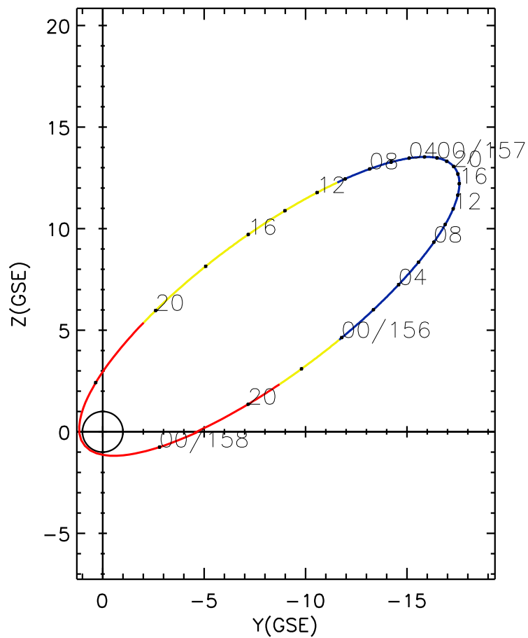
CLUSTER 2 orbit 2024 155 (06/03) 18:31 UT to 2024 158 (06/06) 00:46 UT
