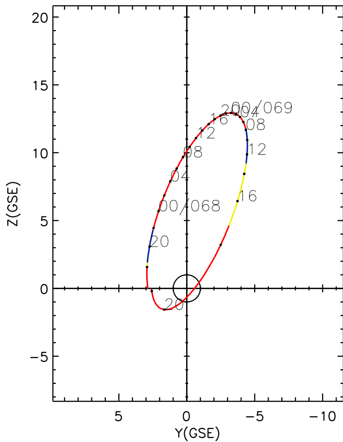
CLUSTER 2 orbit 2024 067 (03/07) 16:01 UT to 2024 069 (03/09) 22:11 UT
