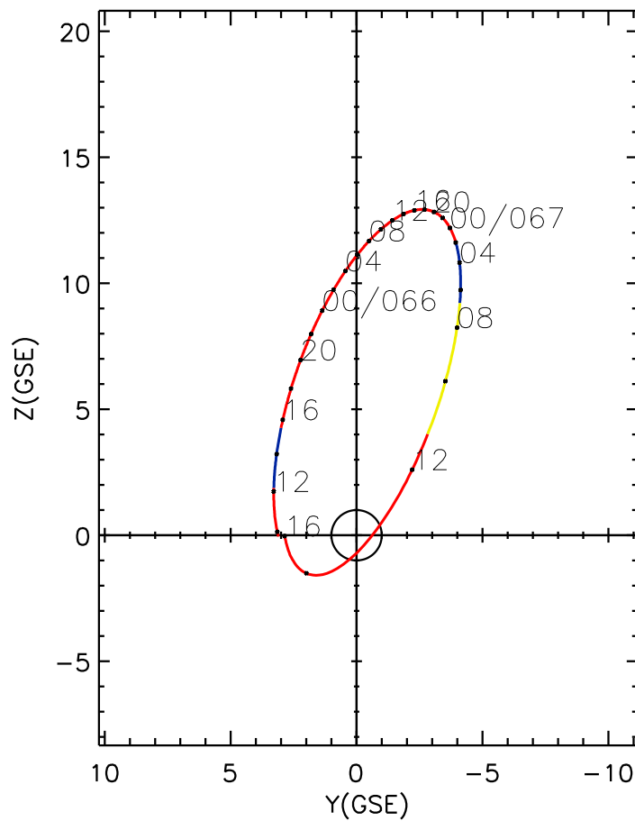
CLUSTER 2 orbit 2024 065 (03/05) 09:46 UT to 2024 067 (03/07) 16:01 UT
