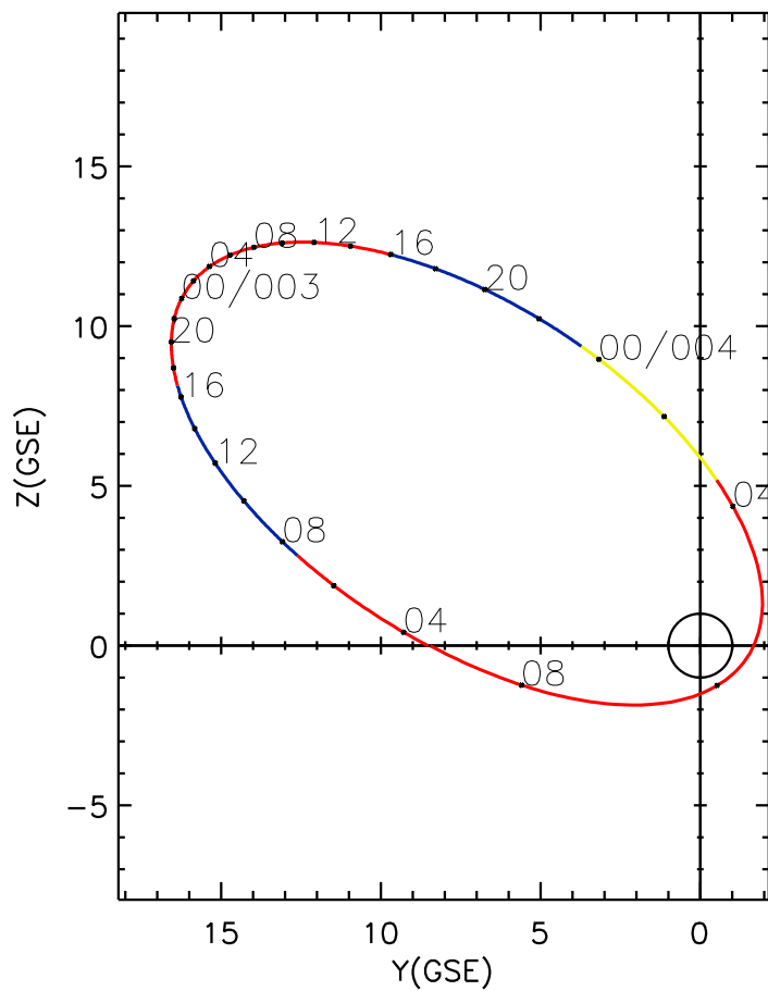
CLUSTER 2 orbit 2024 002 (01/02) 03:26 UT to 2024 004 (01/04) 09:41 UT
