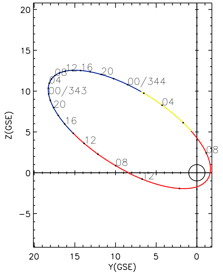
CLUSTER 2 orbit 2023 342 (12/08) 06:46 UT to 2023 344 (12/10) 13:01 UT
