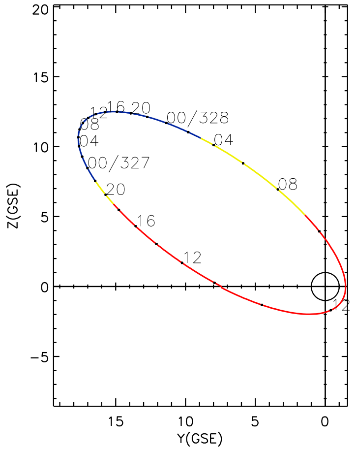
CLUSTER 2 orbit 2023 326 (11/22) 09:36 UT to 2023 328 (11/24) 15:46 UT
