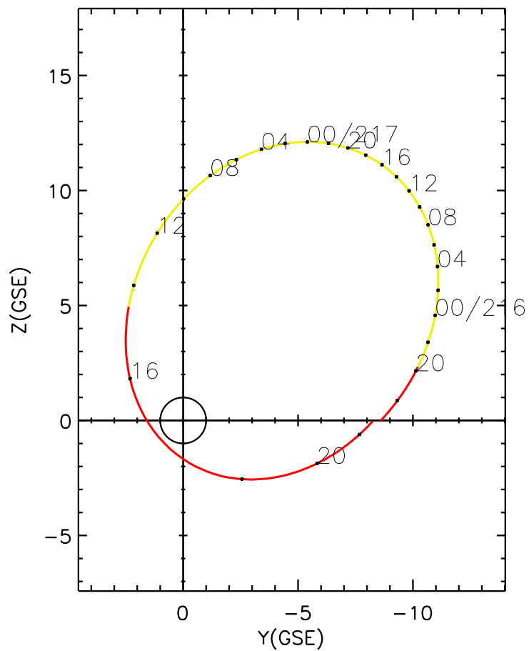
CLUSTER 2 orbit 2023 215 (08/03) 16:41 UT to 2023 217 (08/05) 22:51 UT
