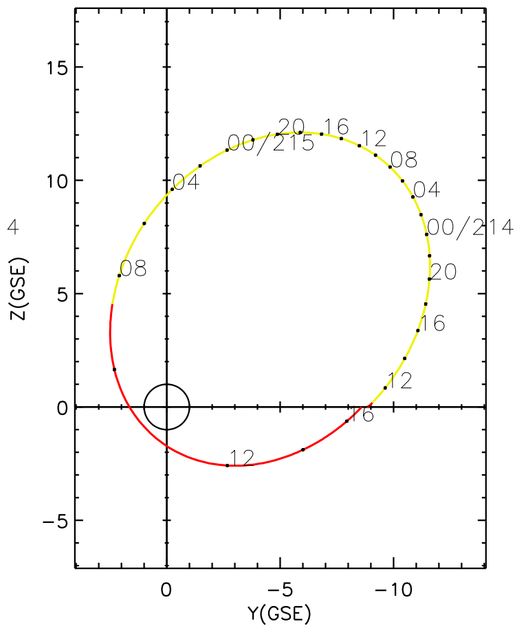
CLUSTER 2 orbit 2023 213 (08/01) 10:41 UT to 2023 215 (08/03) 16:56 UT
