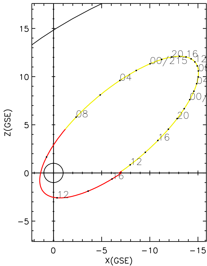
CLUSTER 2 orbit 2023 213 (08/01) 10:41 UT to 2023 215 (08/03) 16:56 UT
