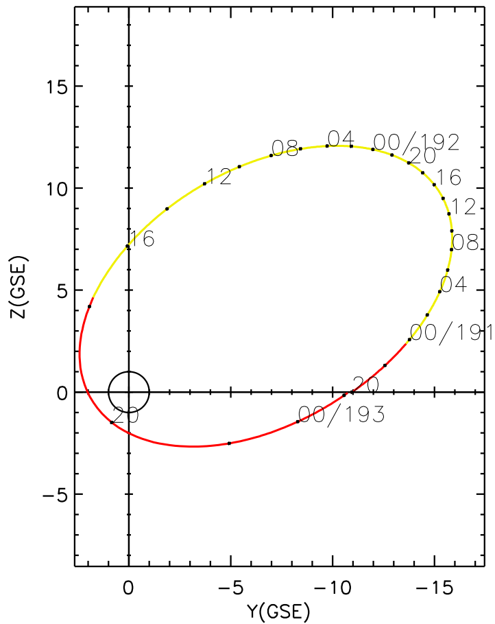
CLUSTER 2 orbit 2023 190 (07/09) 19:56 UT to 2023 193 (07/12) 02:11 UT
