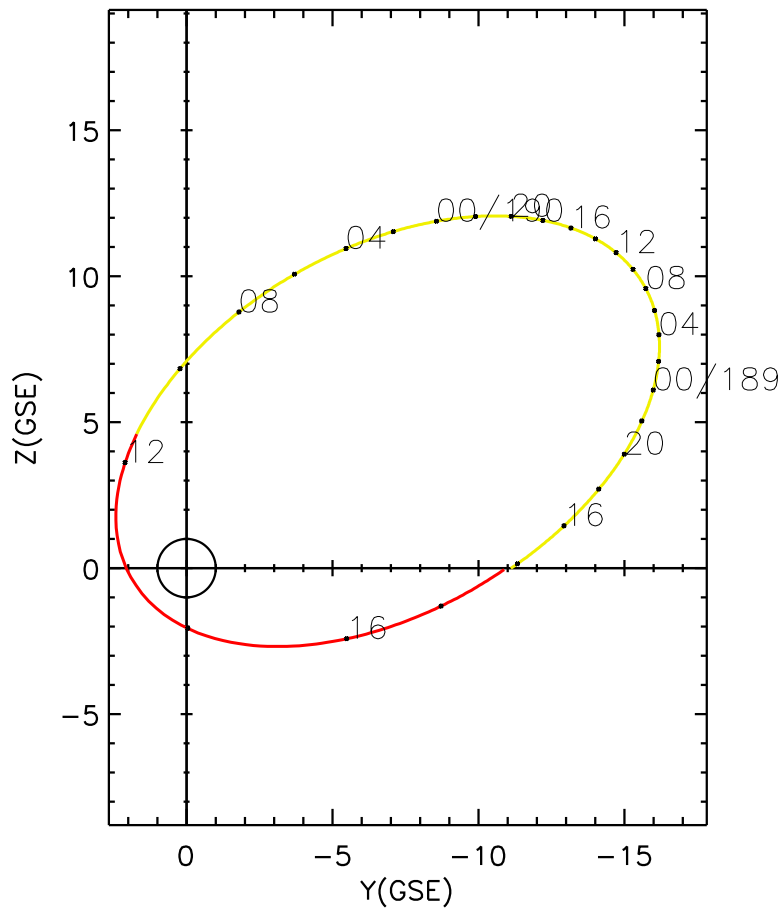
CLUSTER 2 orbit 2023 188 (07/07) 13:46 UT to 2023 190 (07/09) 19:56 UT
