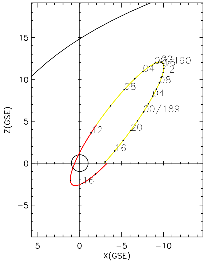
CLUSTER 2 orbit 2023 188 (07/07) 13:46 UT to 2023 190 (07/09) 19:56 UT
