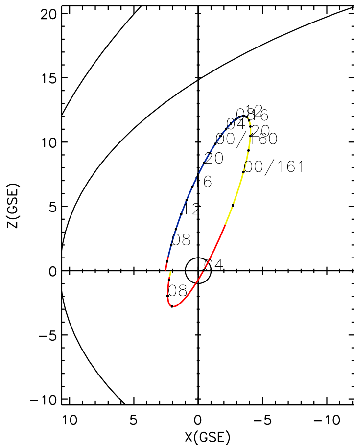
CLUSTER 2 orbit 2023 159 (06/08) 04:51 UT to 2023 161 (06/10) 11:06 UT
