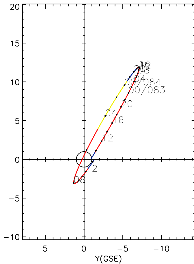
CLUSTER 2 orbit 2023 082 (03/23) 08:16 UT to 2023 084 (03/25) 14:26 UT
