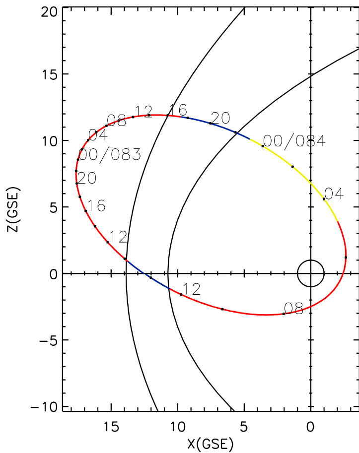
CLUSTER 2 orbit 2023 082 (03/23) 08:16 UT to 2023 084 (03/25) 14:26 UT
