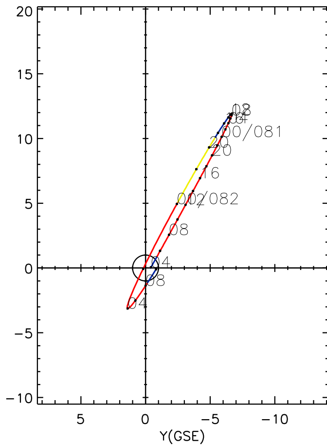
CLUSTER 2 orbit 2023 080 (03/21) 03:51 UT to 2023 082 (03/23) 10:06 UT
