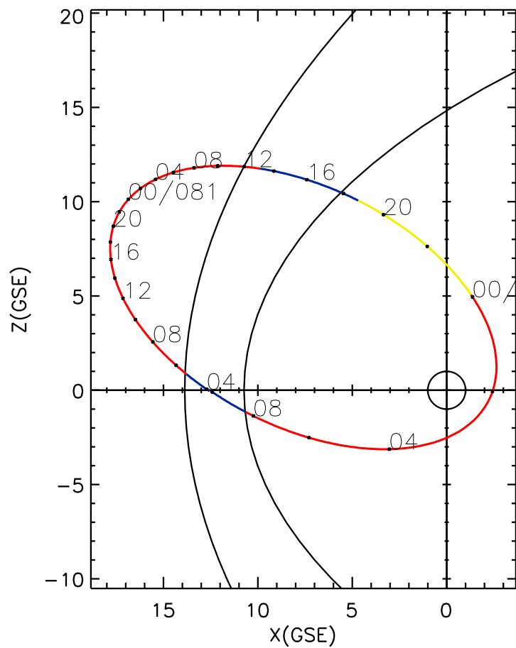
CLUSTER 2 orbit 2023 080 (03/21) 03:51 UT to 2023 082 (03/23) 10:06 UT
