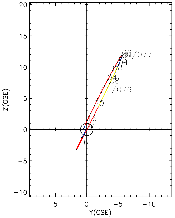
CLUSTER 2 orbit 2023 075 (03/16) 13:46 UT to 2023 077 (03/18) 20:01 UT
