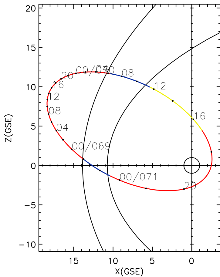
CLUSTER 2 orbit 2023 068 (03/09) 20:41 UT to 2023 071 (03/12) 02:56 UT
